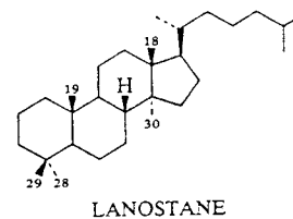
LANOSTANE
