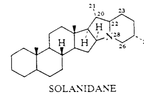
SOLANIDANE
