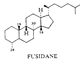
FUSIDANE
