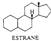
ESTRANE
