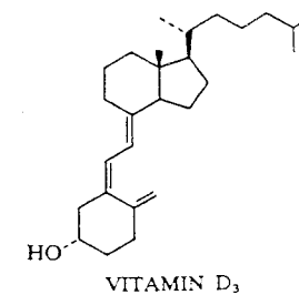
VITAMIN D 3
