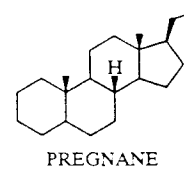
PREGNANE
