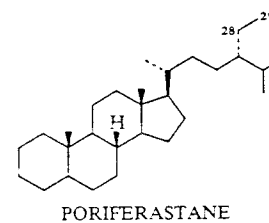
PORIFERASTANE
