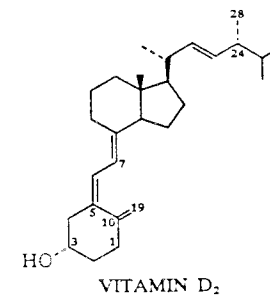
VITAMIN D 2
