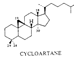
CYCLOARTANE
