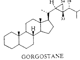
GORGOSTANE
