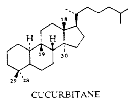
CUCURBITANE
