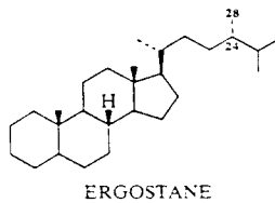
ERGOSTANE
