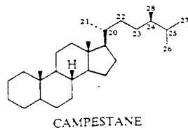
CAMPESTANE
