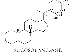
SECOSOLANIDANE
