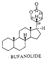
BUFANOLIDE
