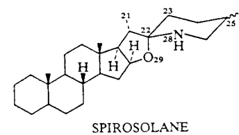
SPIROSOLANE
